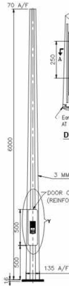
ELEVATION
