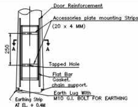
DETAIL Y
